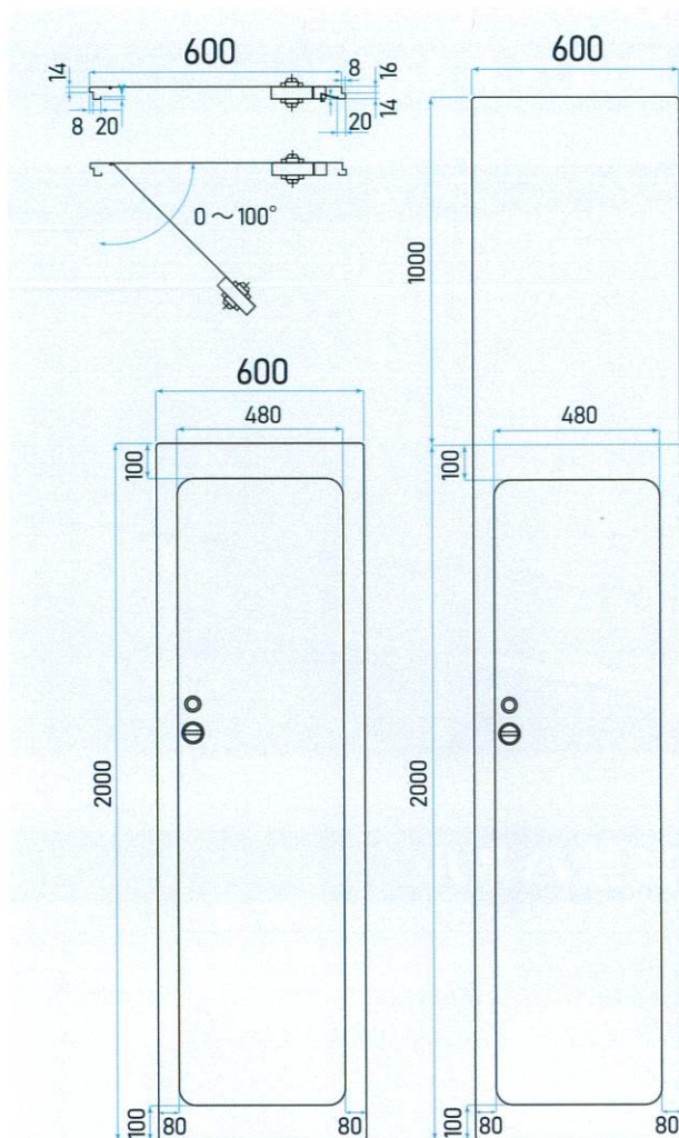
ミニドア
